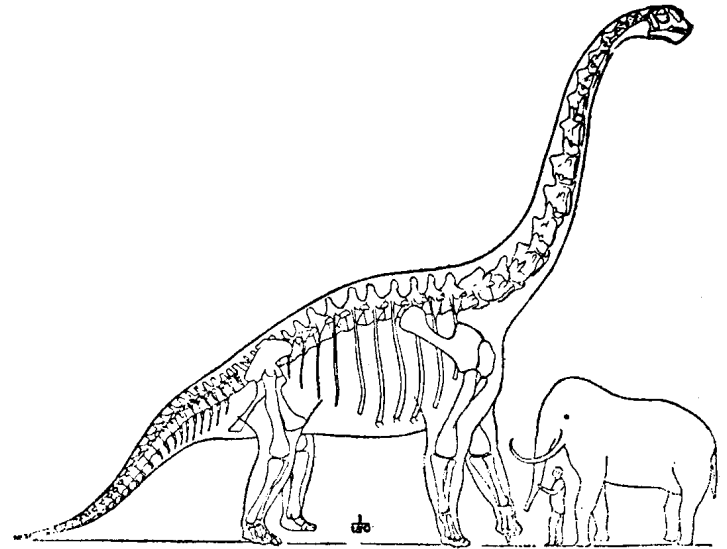
Брахиозаурус (Гигантозаурус), слика 180 пута мања но што је животиња. Оставио је своје кости у Горњој Јури. Тежак је до 4.000 кгр. Сродници су му бронигозаурус и диплодокус. За упоређење дат је поред слона и човека.
