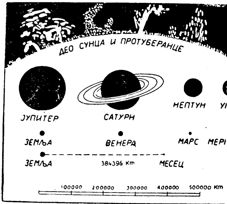
Упоредна величина Сунца, планета и даљине Земља — Месец
