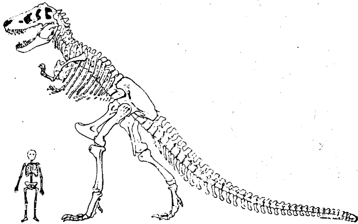
Скелет „Краља тиранозаура” упоређен са скелетом човека (По Осборну)
